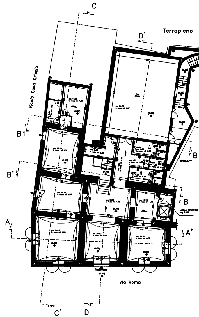
Pianta Architettonica: Livello 0
