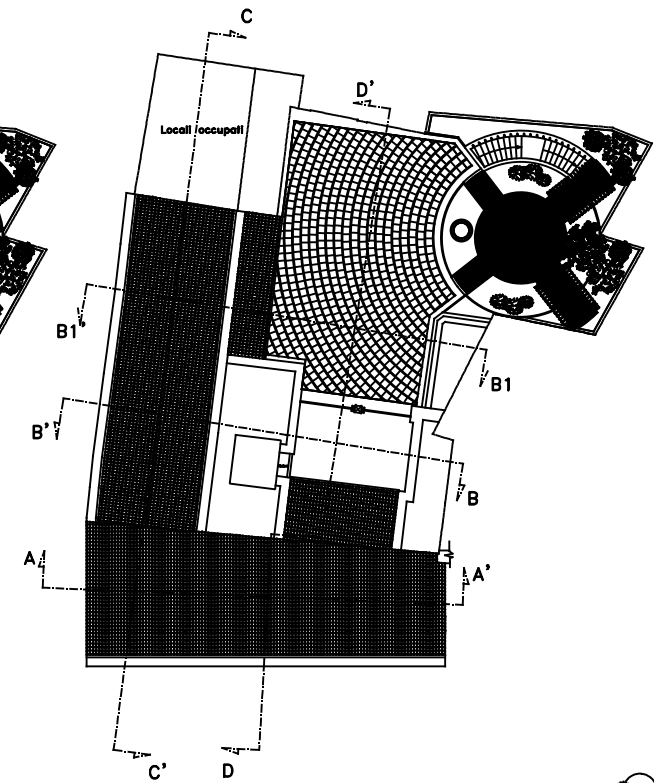
Pianta Architettonica: Coperture
