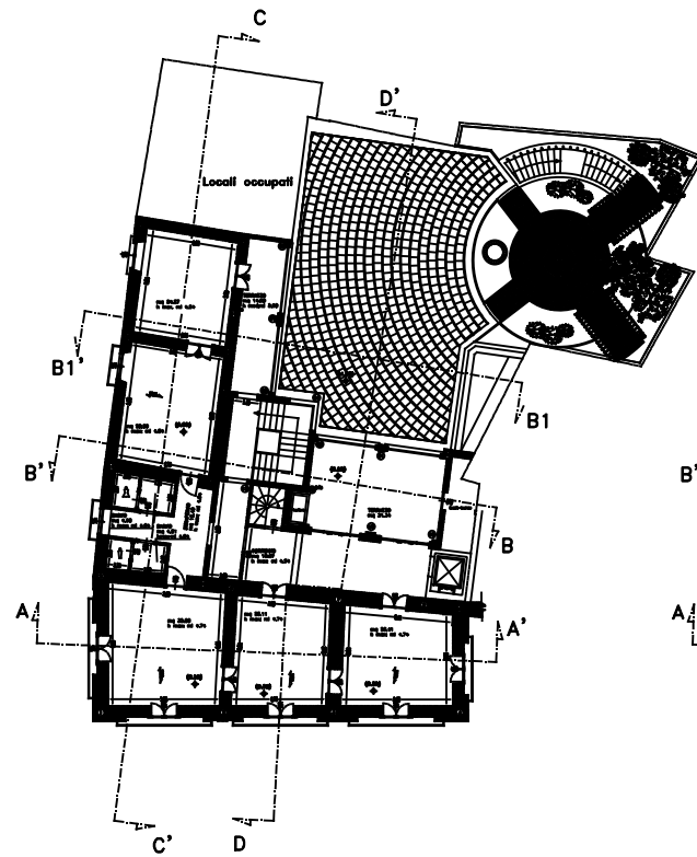
Pianta Architettonica: Livello 2
