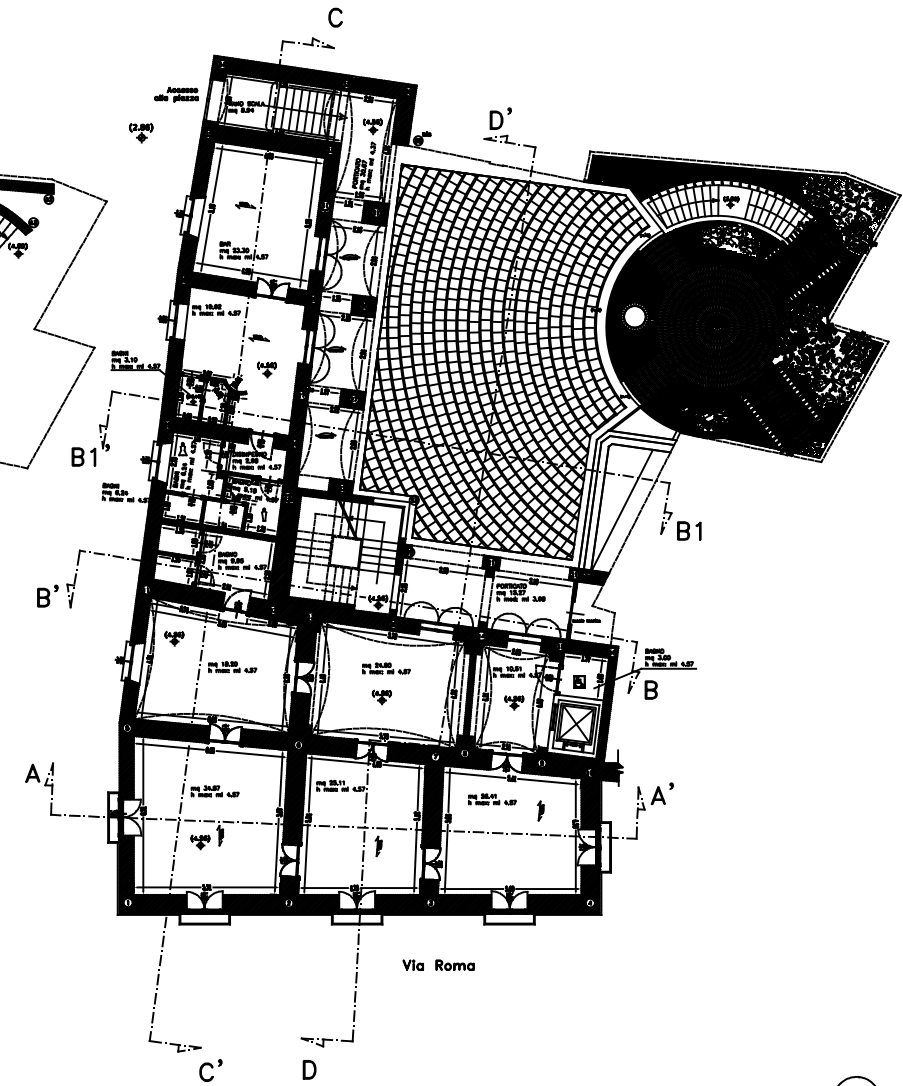
Pianta Architettonica: Livello 1
